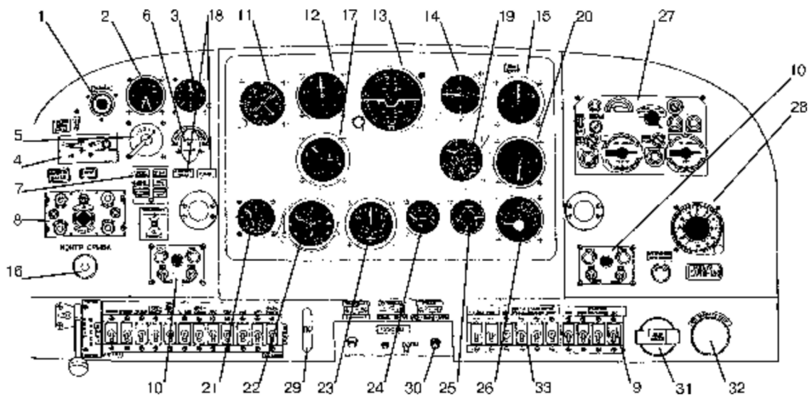
Приборная доска Як-18Т в стандартной комплектации
